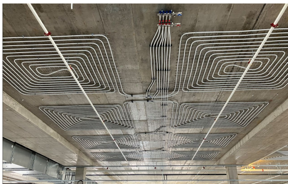
Instalace Klima Panelů pro stropní vytápění / chlazení
