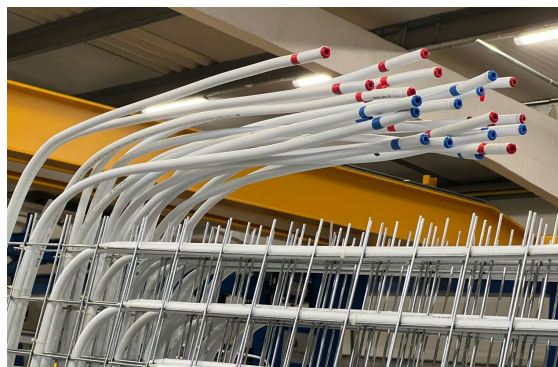
Zaslepení trubek Radopress pro logistiku panelů
