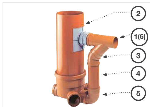
Příklad spadiště na šachtě DN 400
