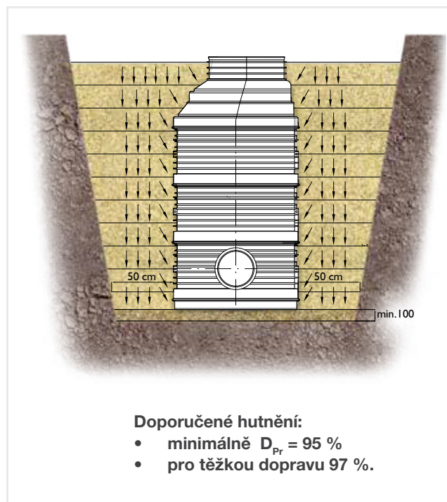
Směry hutnění (platí i pro revizní šachty)
