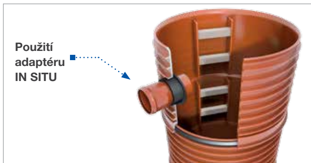
Boční vtok u šachty DN 1000
