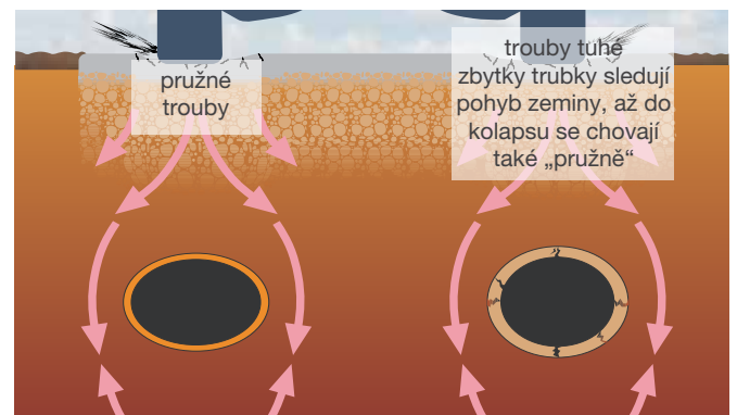
Reakce trubek na zatížení
