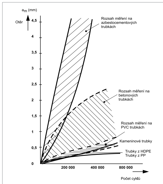
Odolnost vůči abrazi metodou Darmstadt (EN 295-3)
