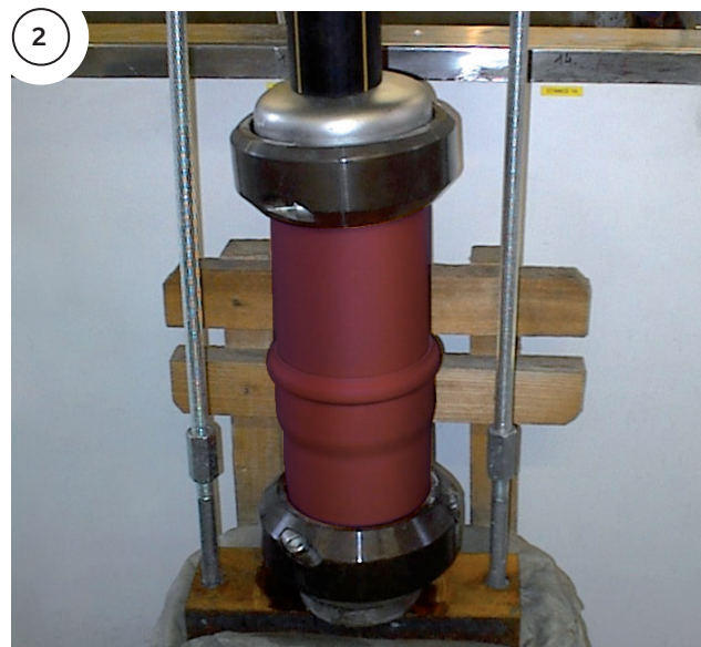
Zkouška těsnosti 2,5 baru
