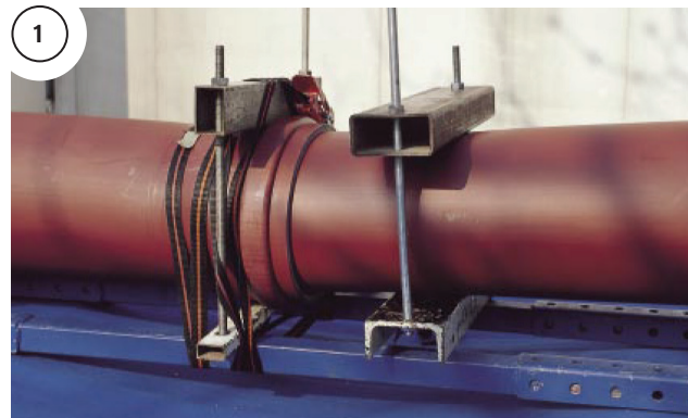
Zkouška těsnosti EN 1277
