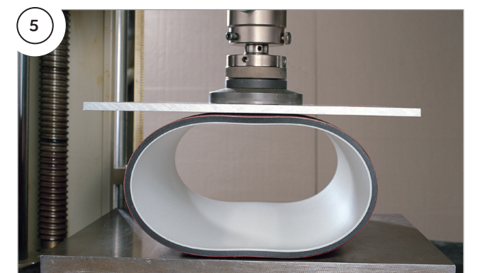
Zkouška kruhové pružnosti
