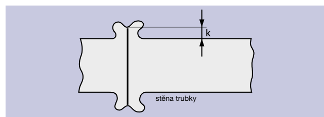
Výška svarového nákrůžku
